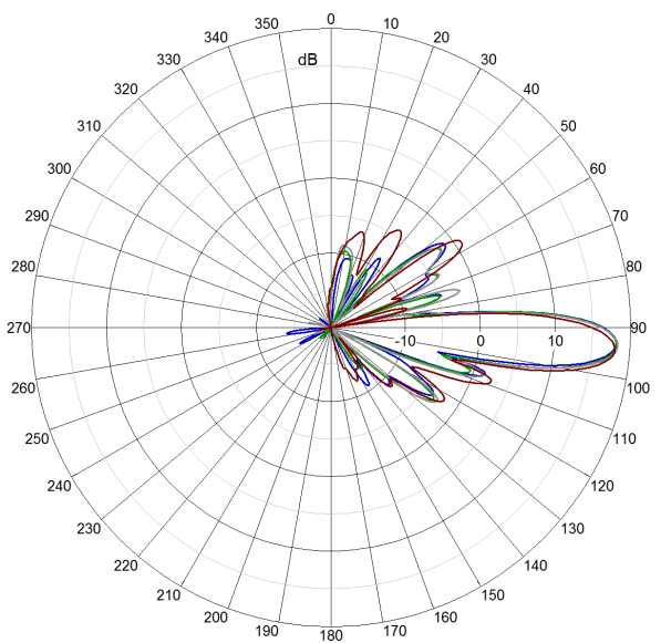
1948 MHz Elevation 4°
